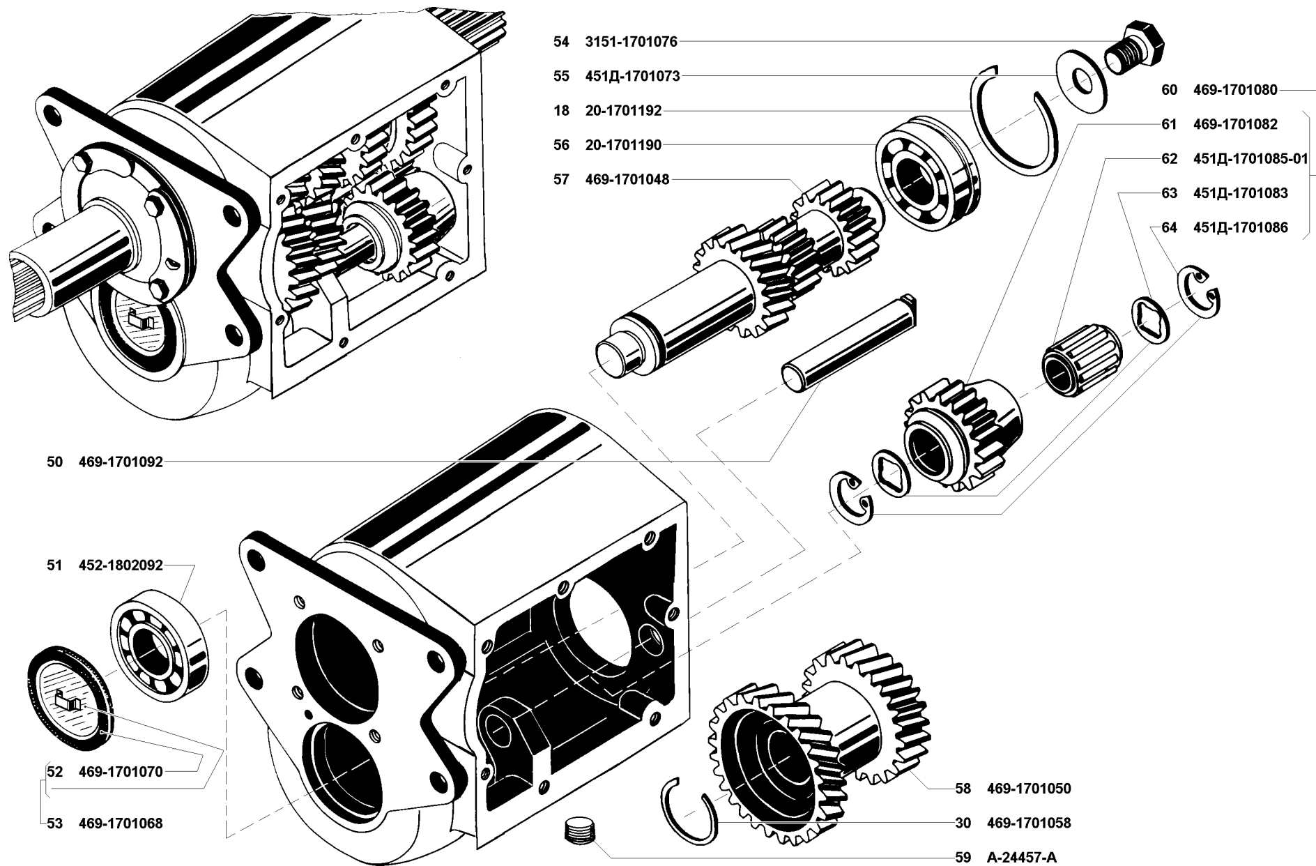
Рис. 45. Коробка передач (1701)/3
